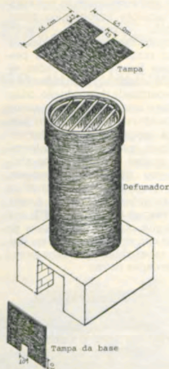
Desenho esquemático do Defumador de Manilha.
